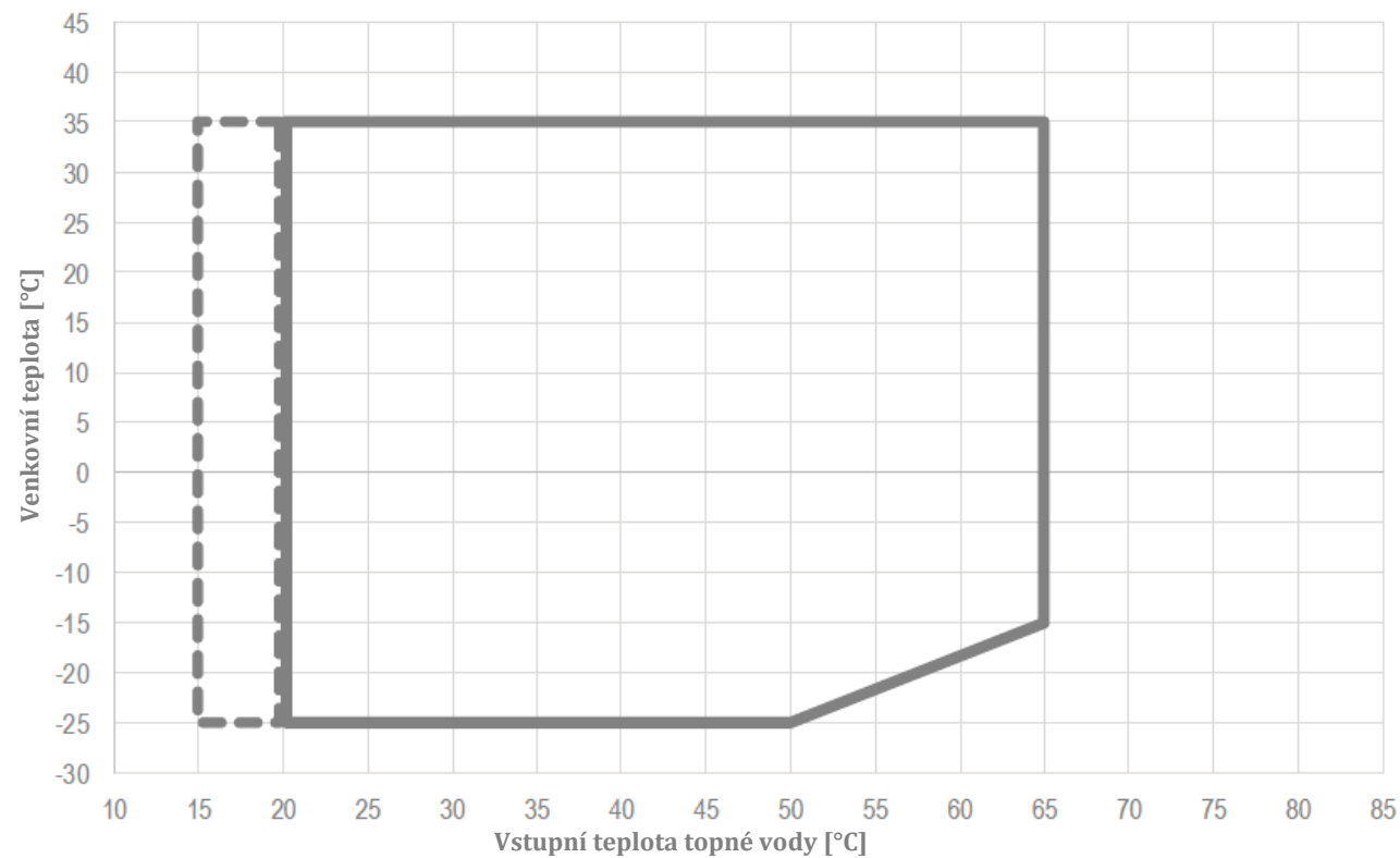
Vstupní teplota
